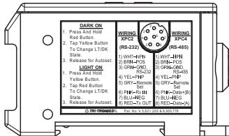
WIRING XPC2 (RS-232)
